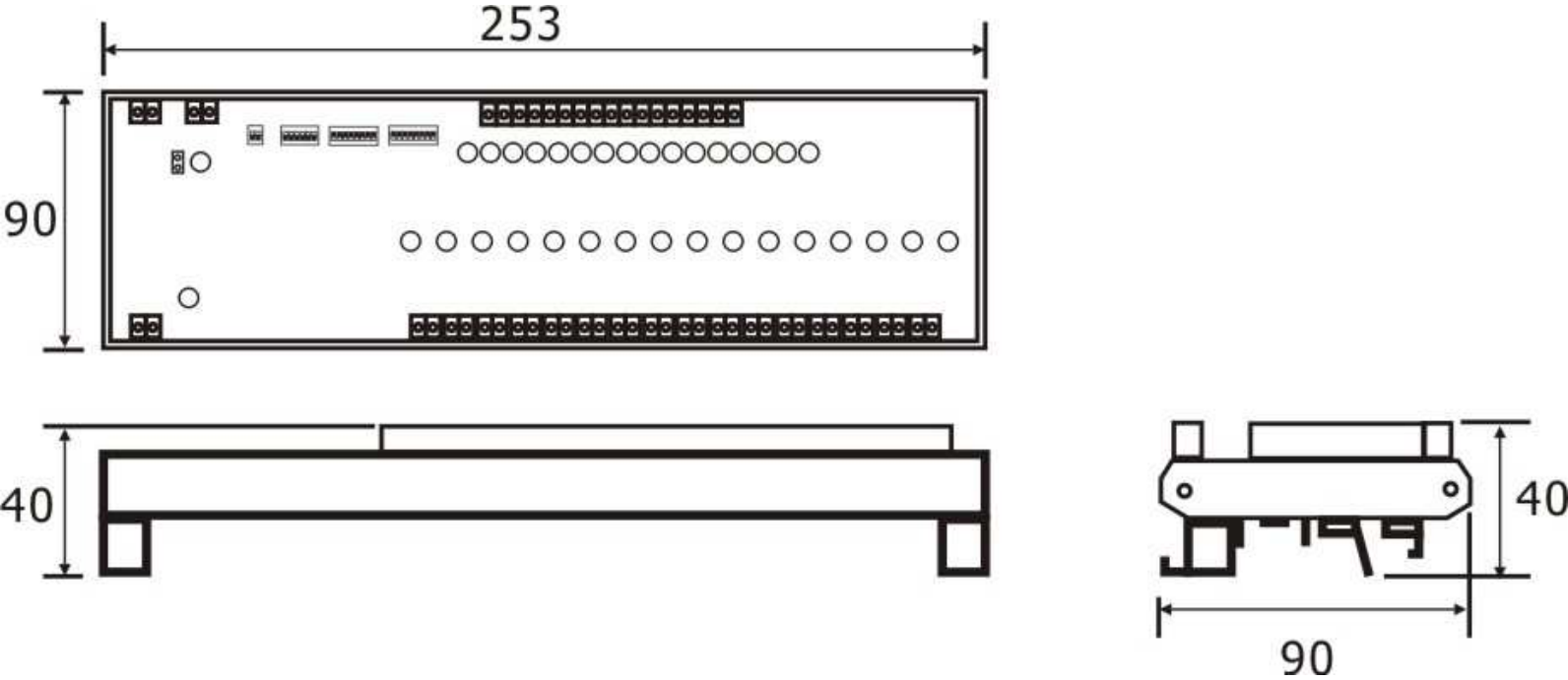
圖 1：IUNT-GEXU 尺寸
